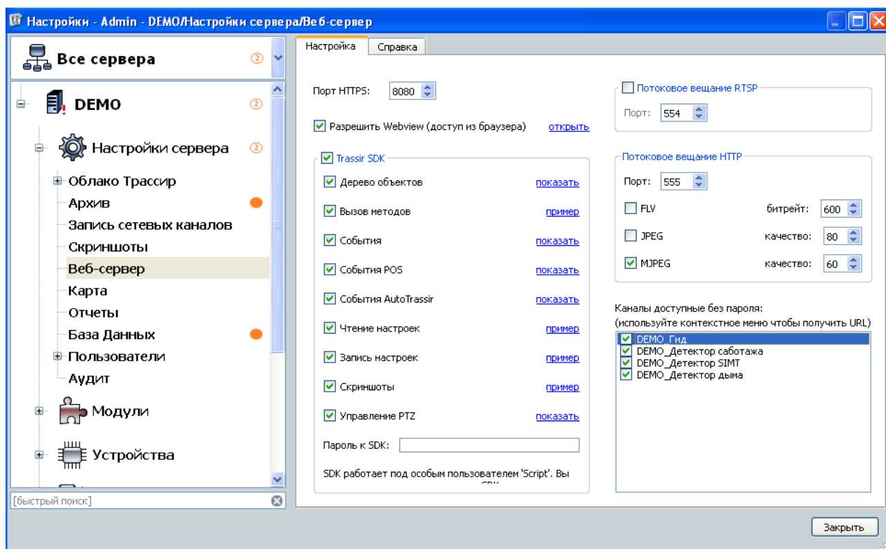
Рисунок 117. Настройки сервера системы видеонаблюдения Trassir 3
